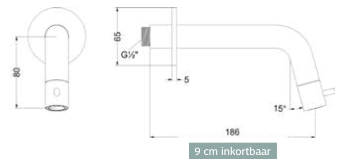
Fonteinkraan wandmodel inkortbaar - Stilo
