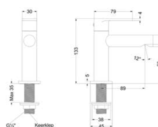
Fonteinkraan staand model S - Forma
