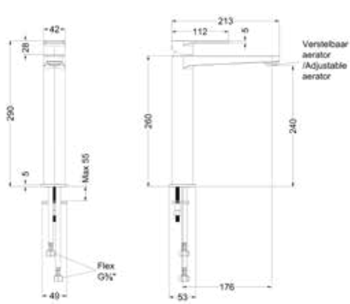
Wastafelmengkraan staand model L - Forma
