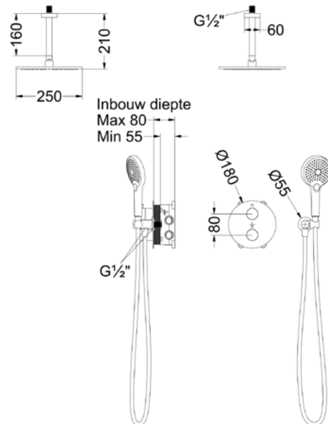
Thermostatische inbouw doucheset - plafondbuis
