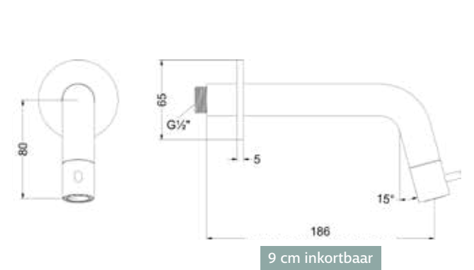
Fonteinkraan wandmodel inkortbaar - Stilo
