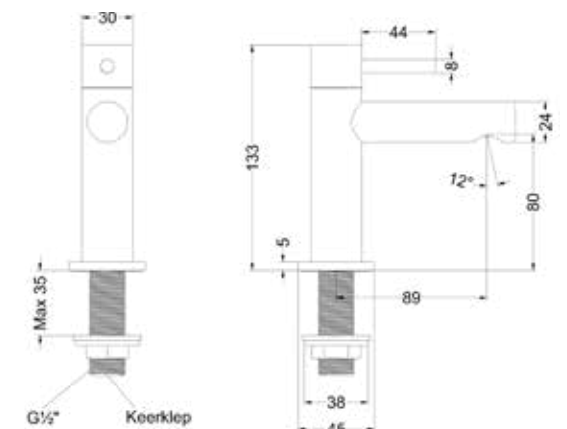
Fonteinkraan staand model S - Stilo
