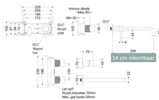
Inbouw wastafelkraan incl. inbouwbox - Stilo
