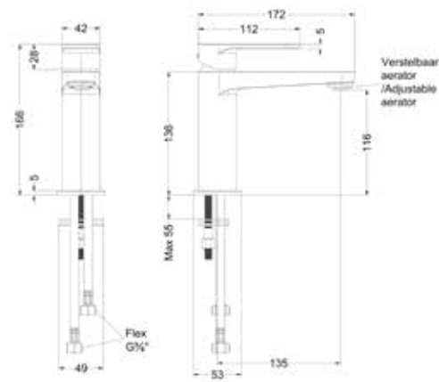
Wastafelmengkraan staand model S - Forma
