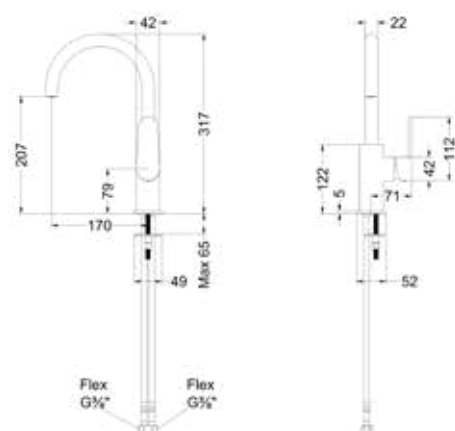
Wastafelmengkraan draaibare uitloop - Forma
